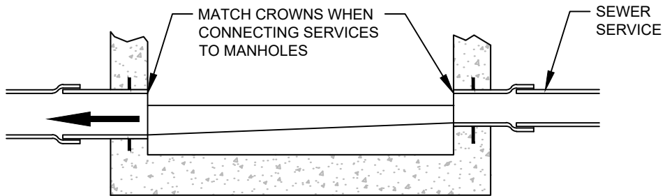
SECTION N.T.S.
