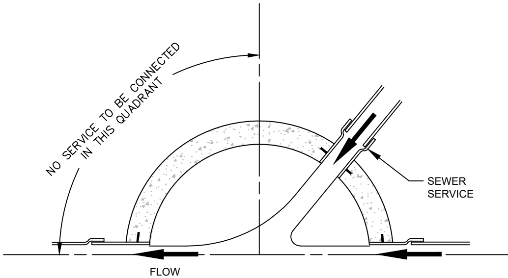
PLAN N.T.S.
