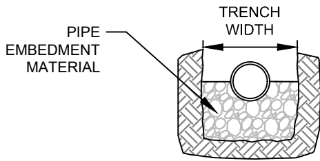
SECTION C-C N.T.S.
