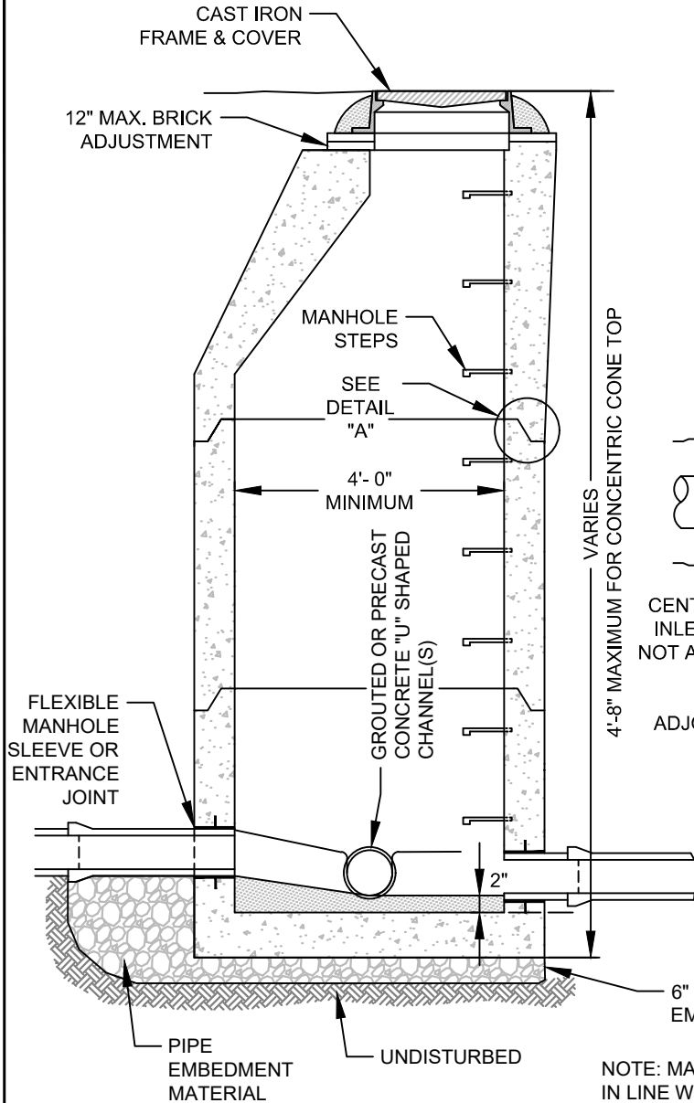
SECTION A-A N.T.S.
