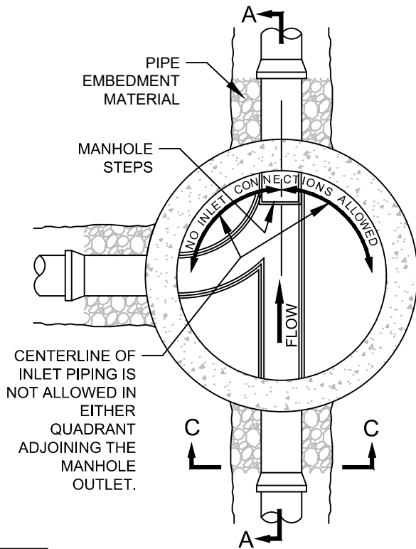
SECTIONAL PLAN N.T.S.
